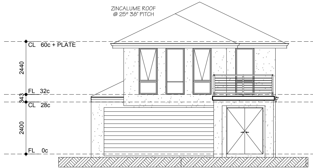
ELEVATION 1 1:100
