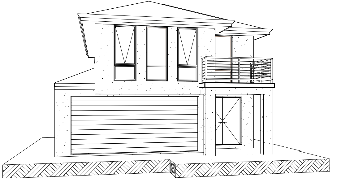
ELEVATION 1 1:100
