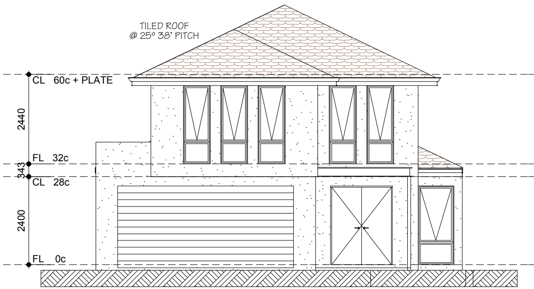
ELEVATION 1 1:100
