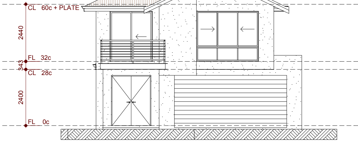
ELEVATION 1 1:100
